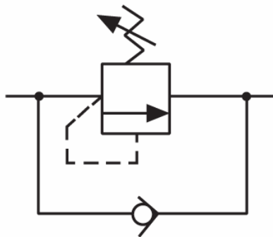
Válvula de contrabalanço com retenção
