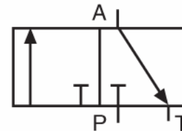
3/2 - NF
