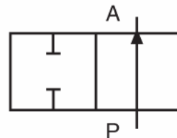
2/2 - NA
