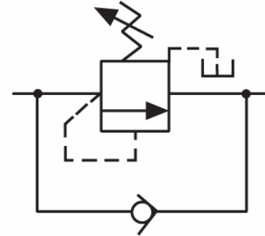
Válvula de sequência com retenção
