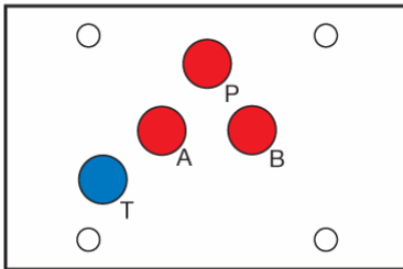
CETOP 5 – TN10
