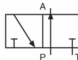
3/2 - NA
